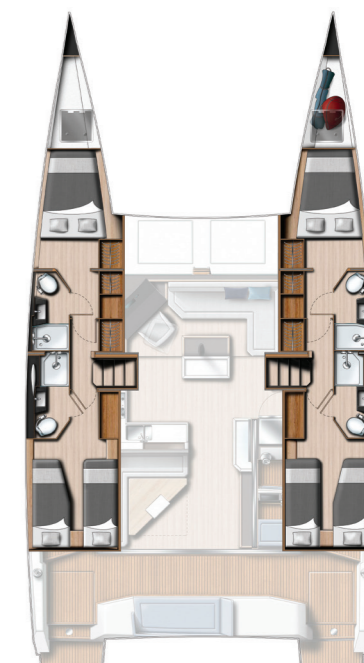
Version 4 Cabines / 4 salles d'eau 4-Cabin / 4-heads version
